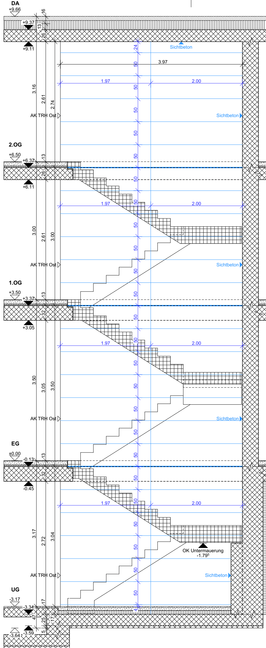
Schnitt TO 2
