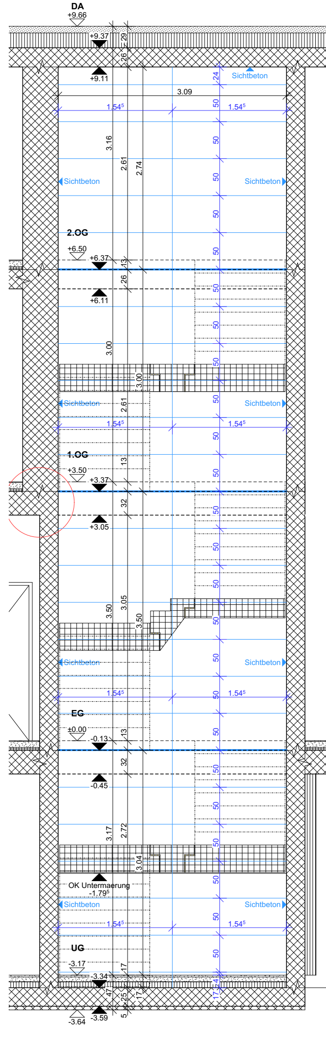
Schnitt TO 4
