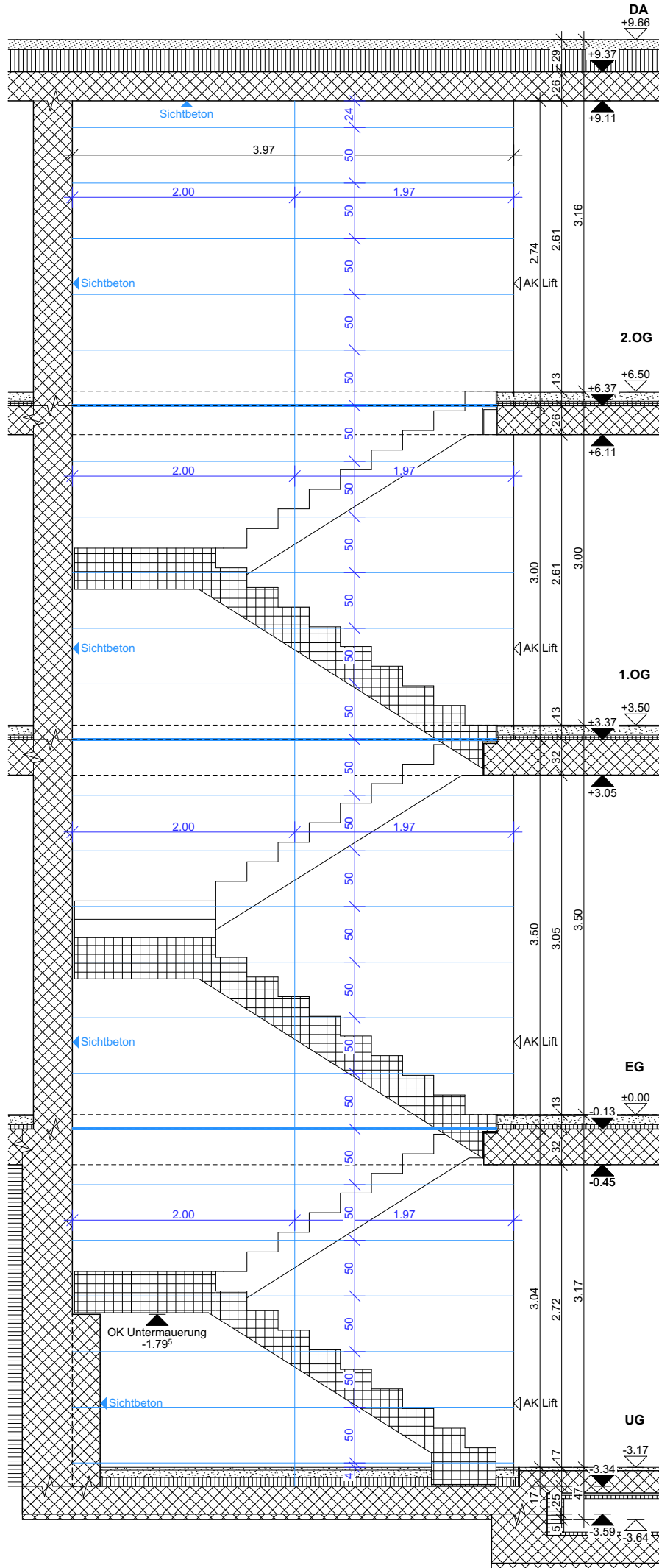
Schnitt TO 1
